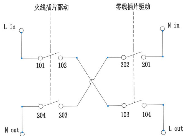
图通领公司插座防触电保护结构原理图
